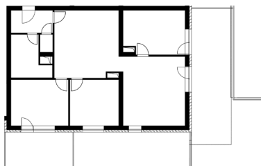
Půdorys bytu (výřez z dokumentace)
